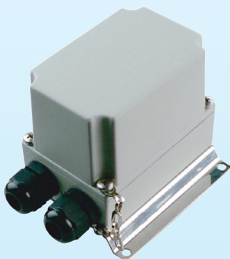
Esempio di montaggio su due cavi di tracciamento del calore di un Y1B2P, in combinazione con la scatola di connessione Y29
